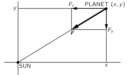
图 9.5: 作用在行星上的太阳引力
